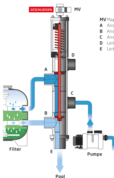
FILTRATIONSMODUS Magnetventil geschlossen
