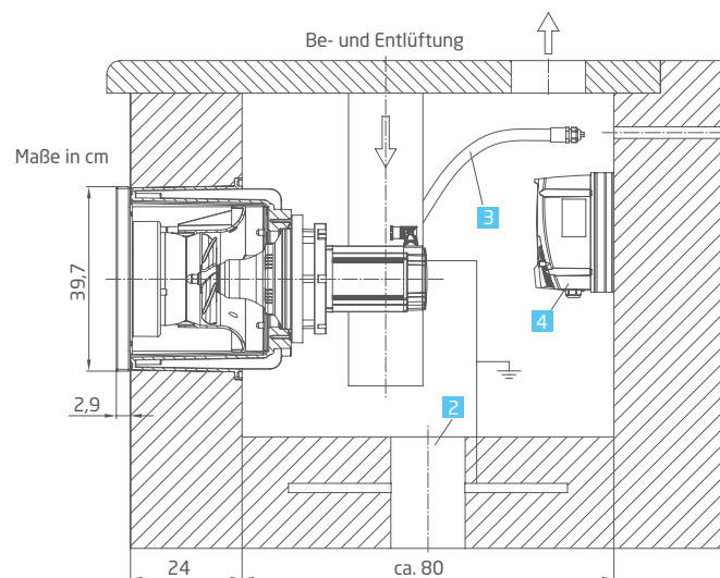
Unverbindliches Einbauschema
