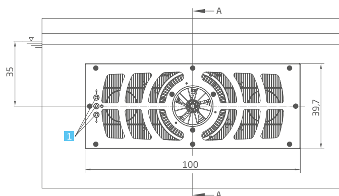
Unverbindliches Einbauschema
