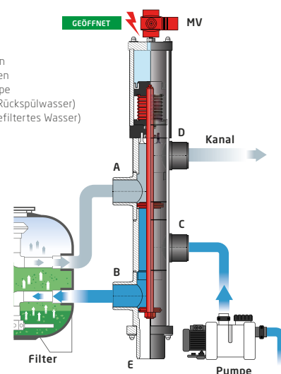
RÜCKSPÜLMODUS Magnetventil geöffnet
